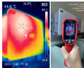
inverter No.4 อุณหภูมิ 46.2 °C
