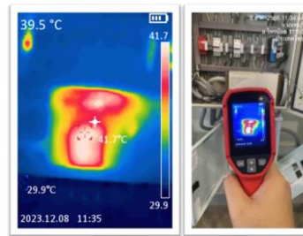
ความร้อน USP 41.7 °C
