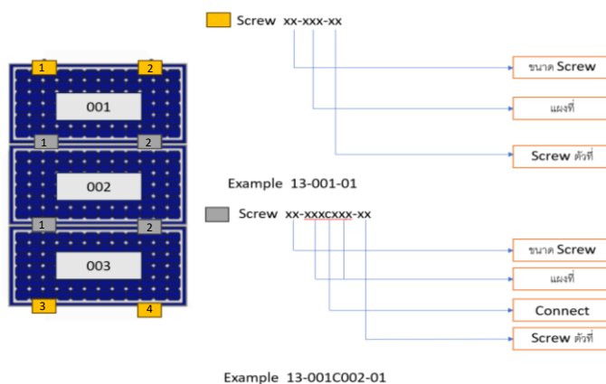
Torque screw ขนาด 13 mm. และขนาด 17 mm.
