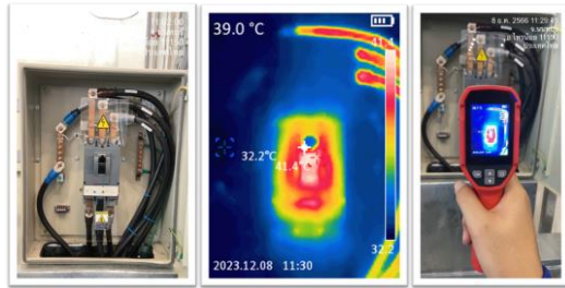
อุณหภูมิ MCCB Cabinet No.2 41.4 °C
