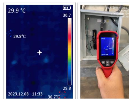
ภายในตู้LP 30.7 °C
