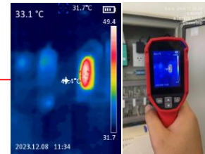
RTU FAN 49.4 °C พัดลมทำงานปกติ
