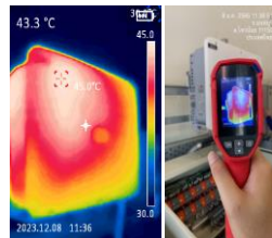
inverter No.3 อุณหภูมิ 45.0 °C
